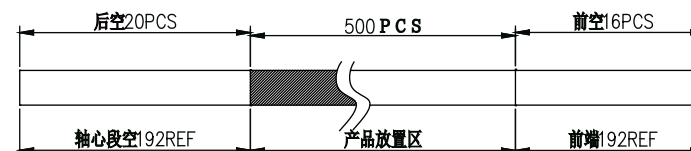
包装示意图:
