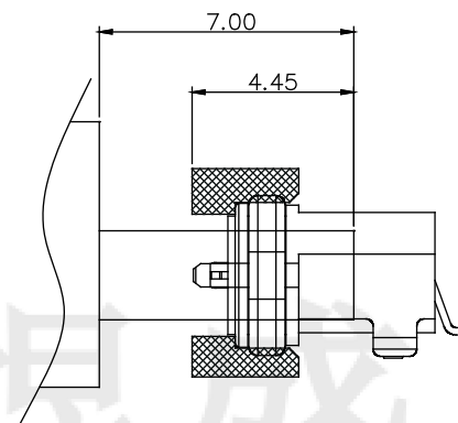
plug插入深度参考图
