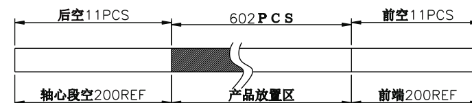
包装示意图:
