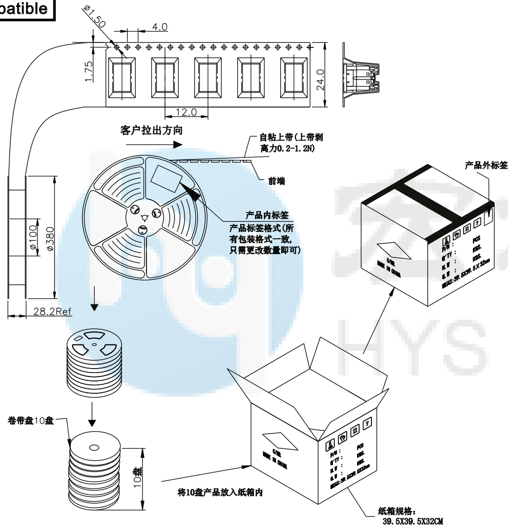
包装示意图:
