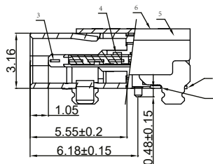
SECTION A-A(剖视图A-A) SCALE 2:1 (比例 2:1)
