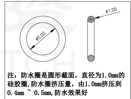
加防水圈示意图
