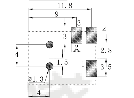
线路板开孔尺寸
