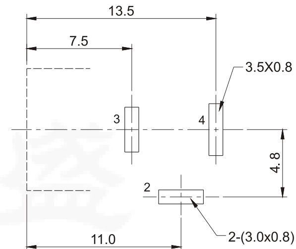
线路板印制示意图
