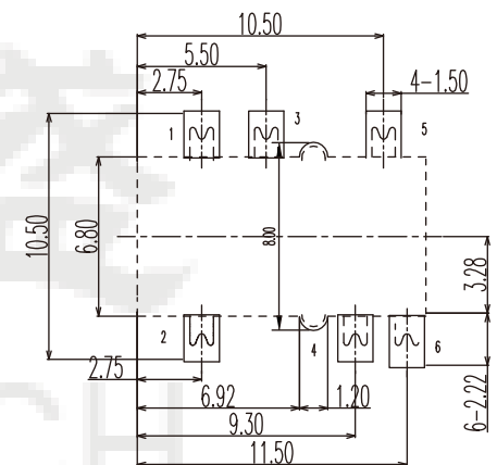
P.C.B LAYOUT TOP VIEW 反貼
