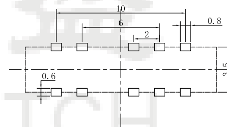
PCB板位置尺寸
