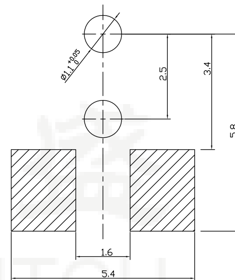
安装位置图
