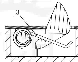
安装位置图
