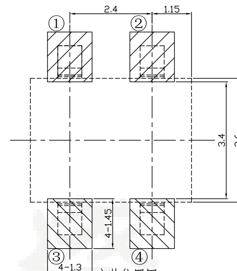
安装位置图
