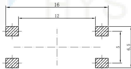
PCB线路板安装图(±0.1)
