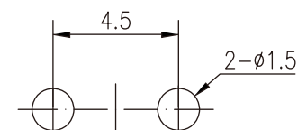
PCB线路板安装图(±0.2)
