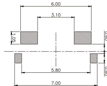
PCB. 焊接图
