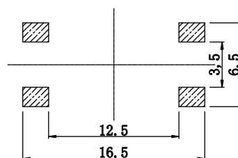
PCB. 焊接图
