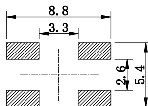
PCB. 焊接图
