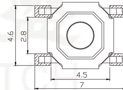
PCB板焊盘尺寸
