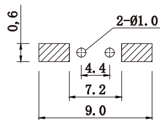
PCB. 焊接图
