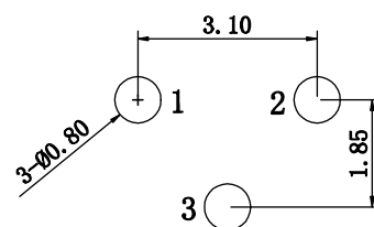
PCB. 焊接图
