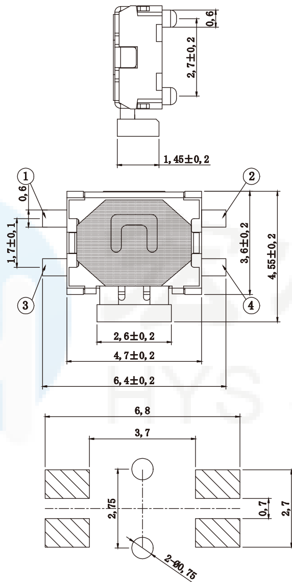
PCB. 焊接图
