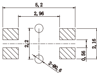
PCB. 焊接图
