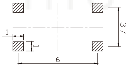
PCB. 焊接图
