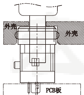
组装示意图
