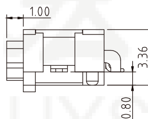
组装示意图
