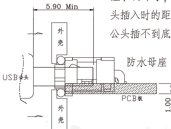
组装示意图
