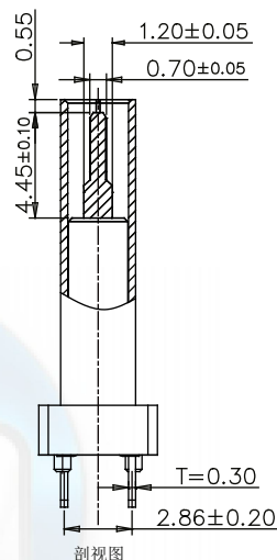
剖视图
