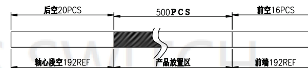
包装示意图:
