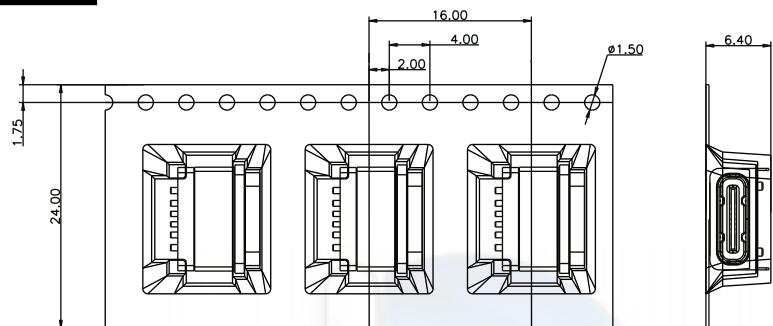
① 产品入载带示意图
