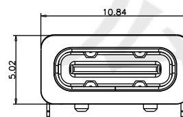
加防水圈示意图
