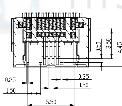
截面 A-A 比例 4:1
