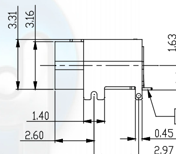
截面 A-A 比例 4:1
