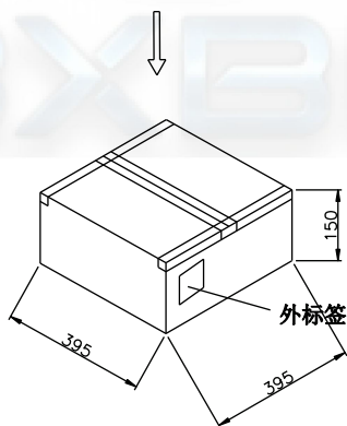
⑤ 外箱封箱示意图
