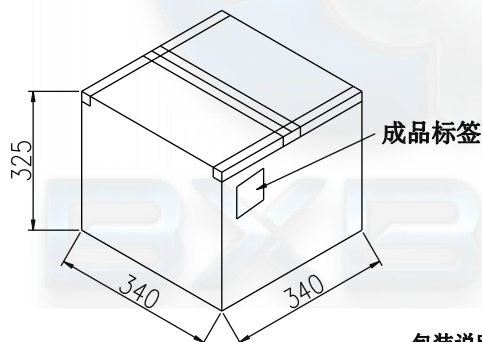
⑤ 外箱封箱示意图
