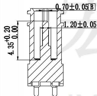
截面A-A
