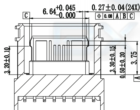
截面B-B
