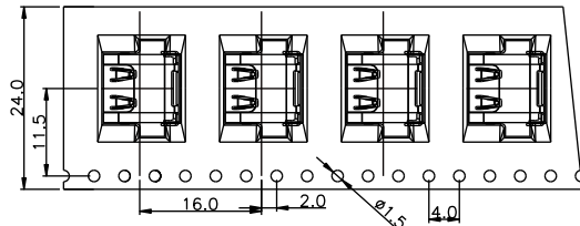
① 产品入载带示意图
