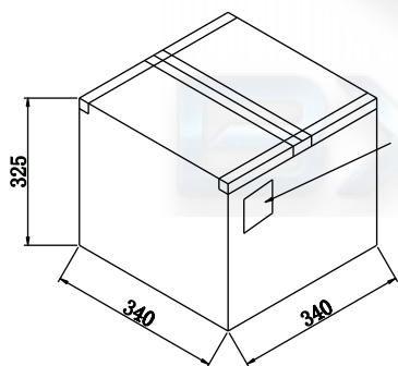
⑤ 外箱封箱示意图
