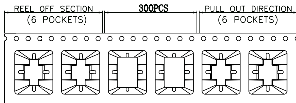
① 产品入载带示意图
