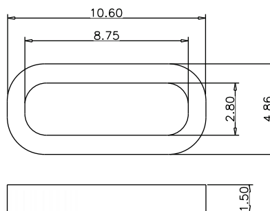
防水圈尺寸图
