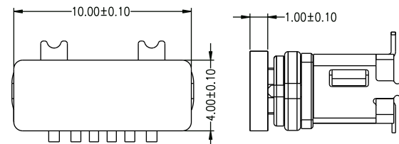
Cap dimensions
