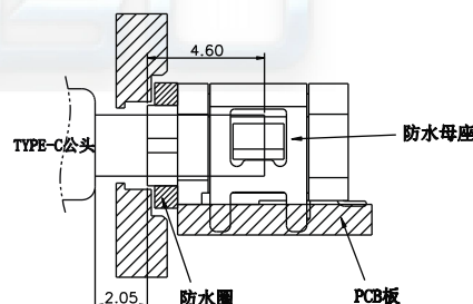
组装示意图 参考图
