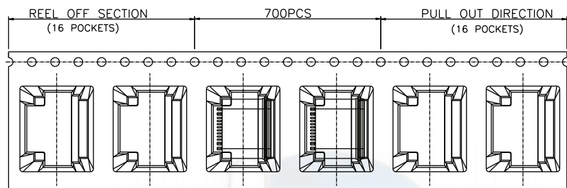
① 产品入载带示意图
