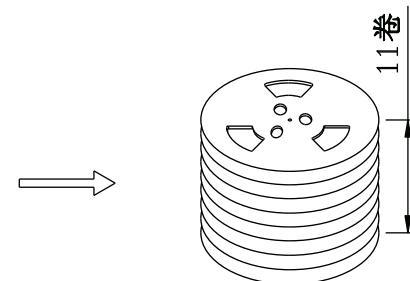
③ 11盘产品叠层示意图
