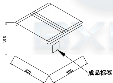
⑤ 外箱封箱示意图
