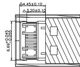
截面A-A
