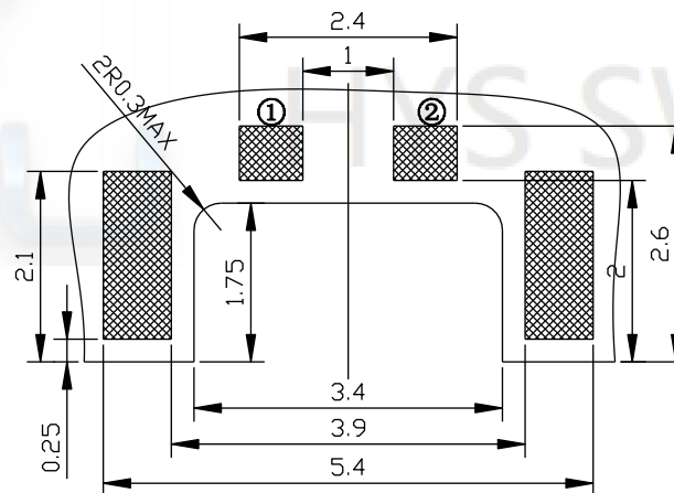
P. C. B 焊接图
