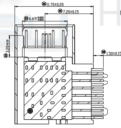
剖视图
