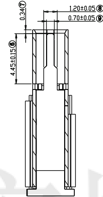
剖视图
