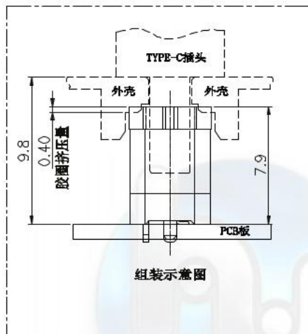
组装示意图
