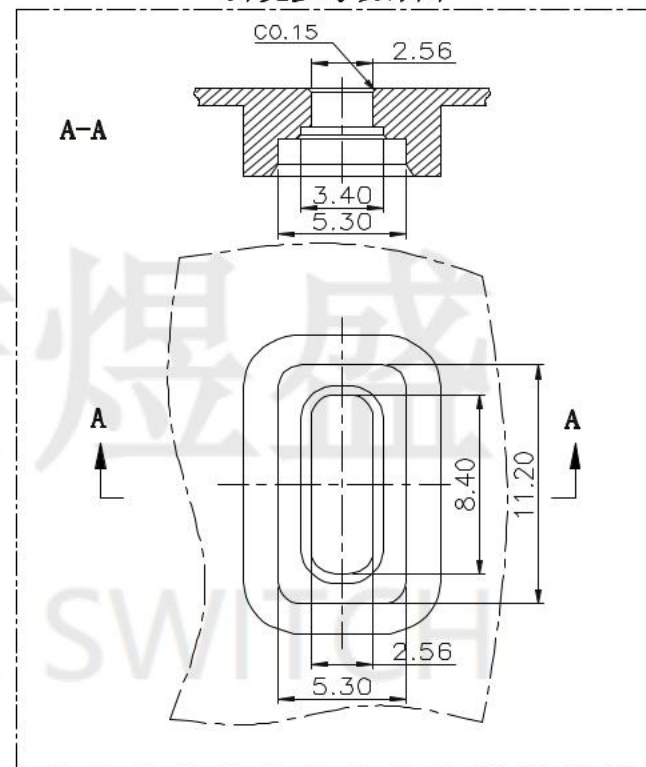
外壳参考设计图
