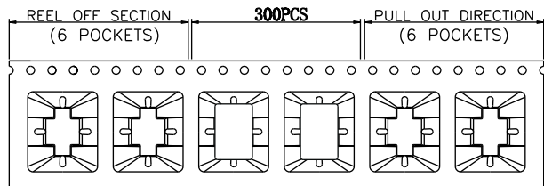
① 产品入载带示意图
