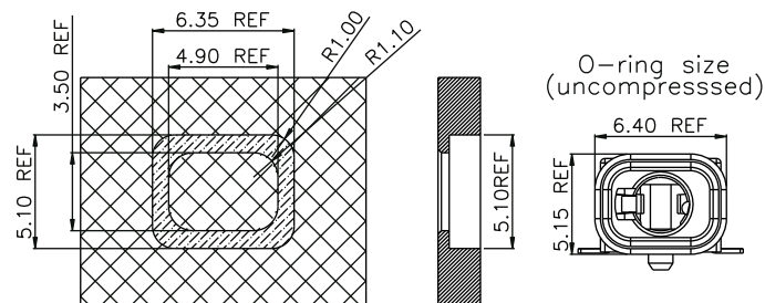
面板开孔参考尺寸
