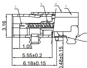
SECTION A-A(剖视图A-A) SCALE 2:1 (比例 2:1)
