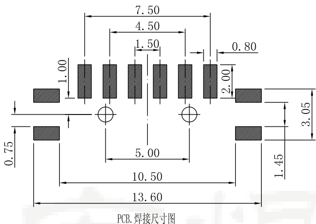
PCB. 焊接尺寸图
